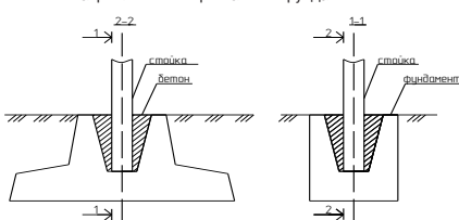
Рис. 1 Закрепление опор знаков в фундаменте
