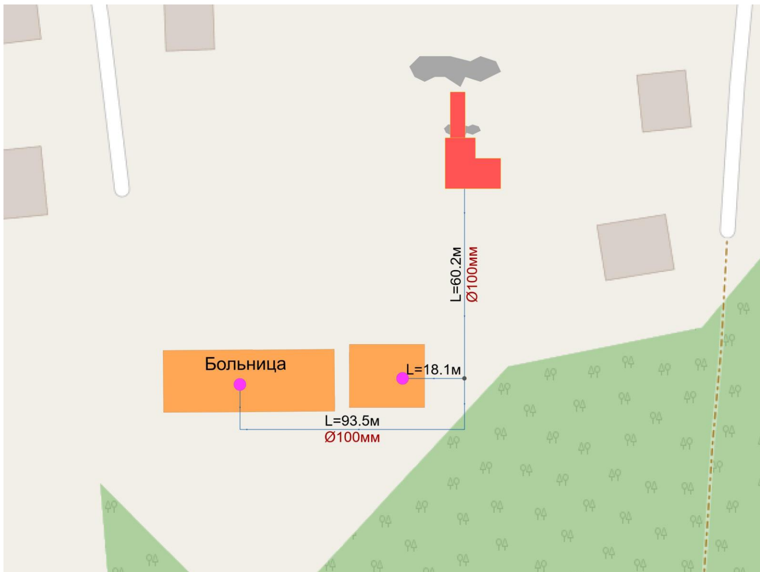
Рис. 2 – Схема теплоснабжения Котельной больницы ул. ЛЗС, 3Ж
