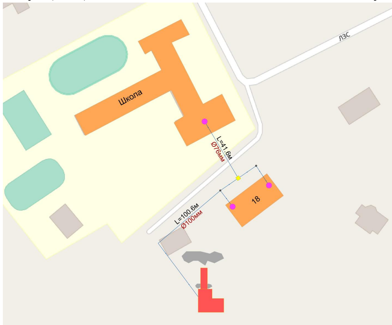
Рис. 1 – Схема теплоснабжения Котельной школы, ул. Школьная, 1Ж
